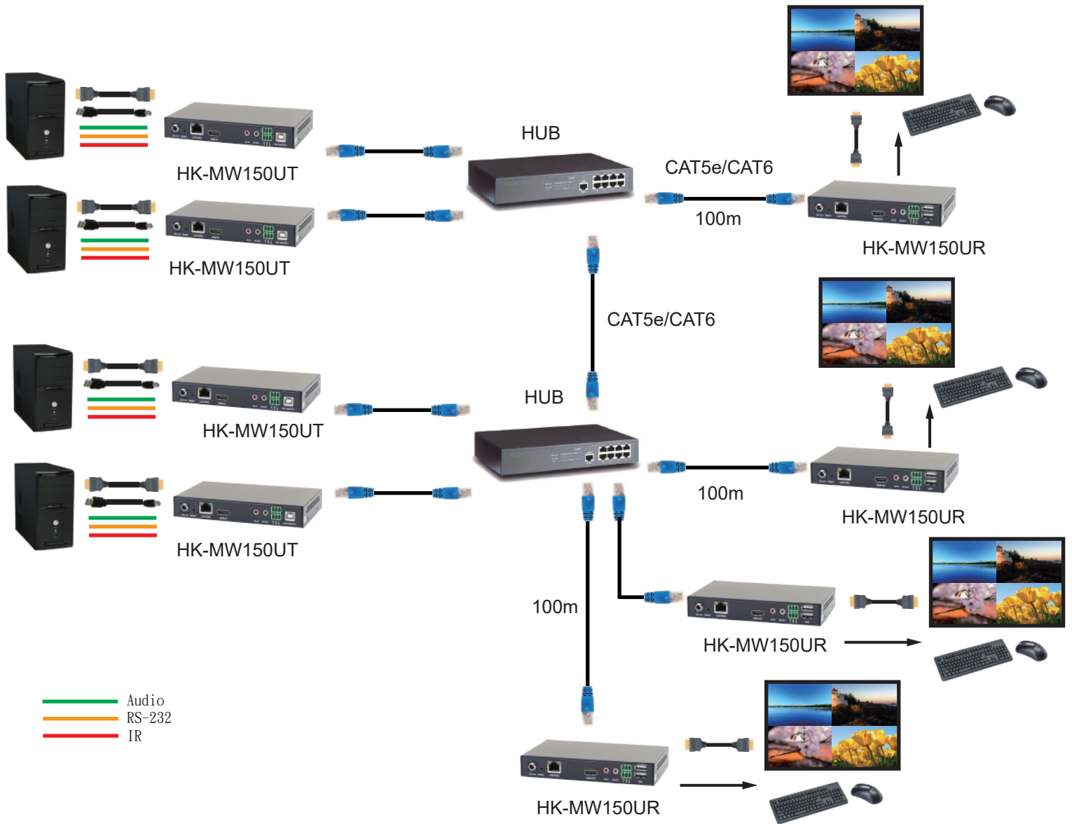
連接示意圖五 ( 多對多 畫面分割 ).
