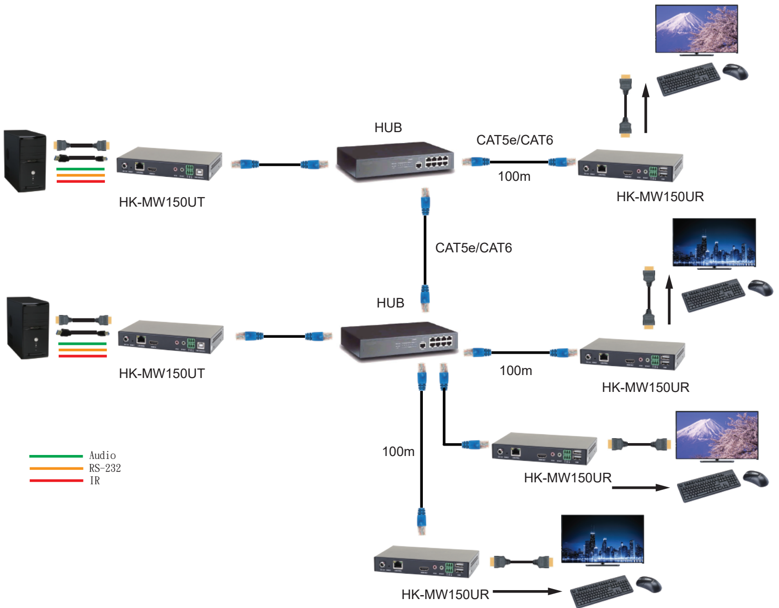
連接示意圖三 ( 多對多 Over LAN ) .
