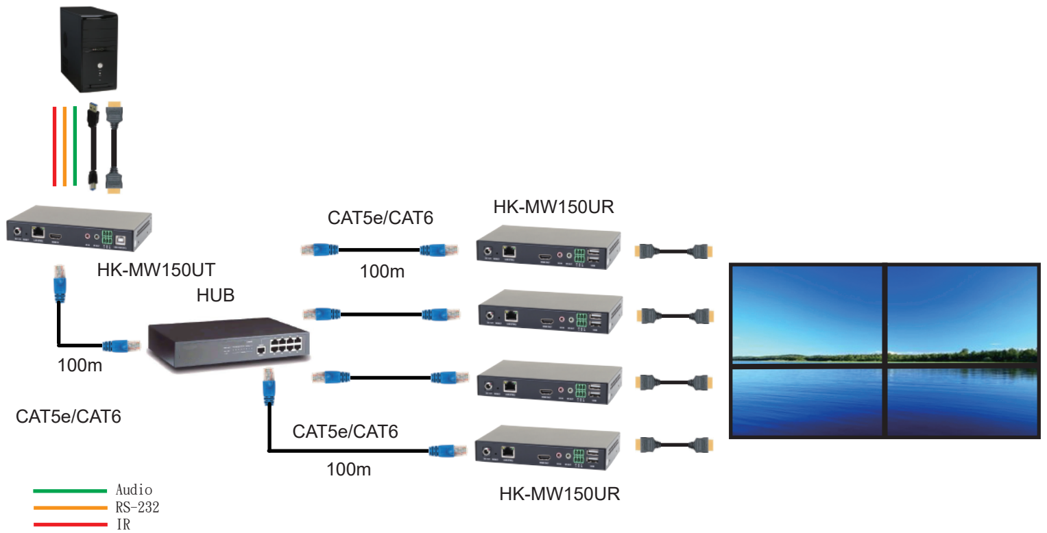
連接示意圖四 ( 1對多 電視牆模式 ).
