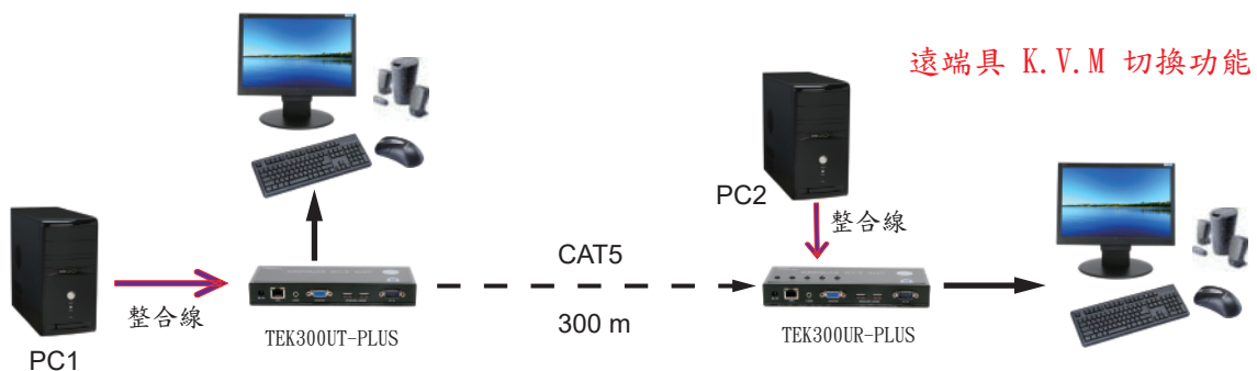
連接示意圖
