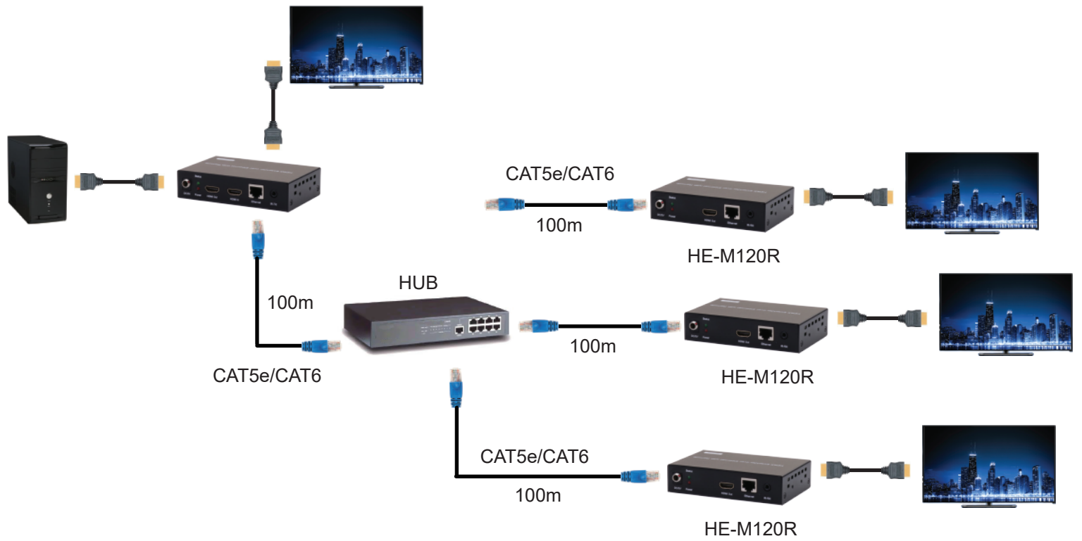
連接示意圖三 ( 多對多 Over LAN ) .
