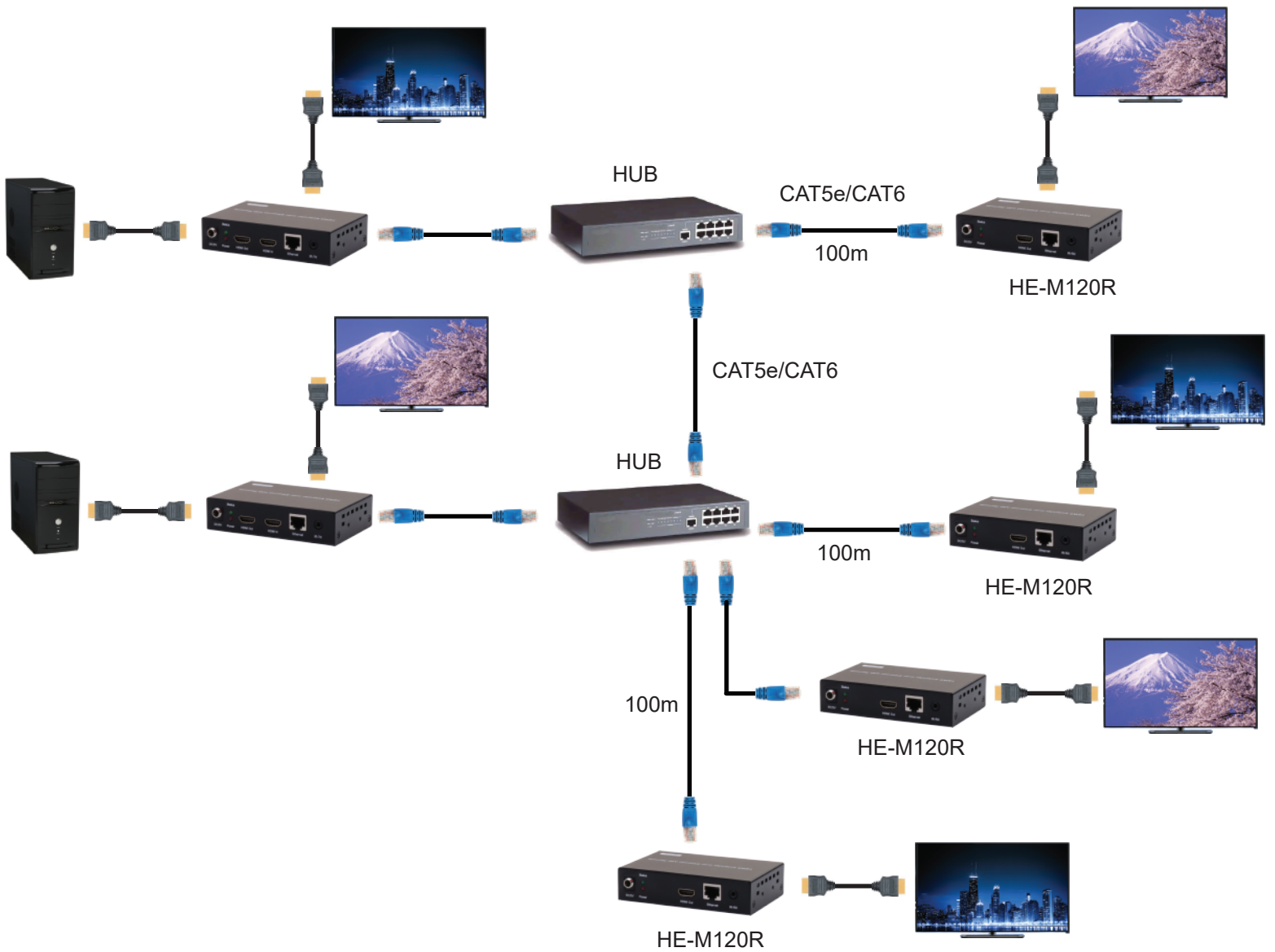
連接示意圖三 ( 多對多 Over LAN ) .
