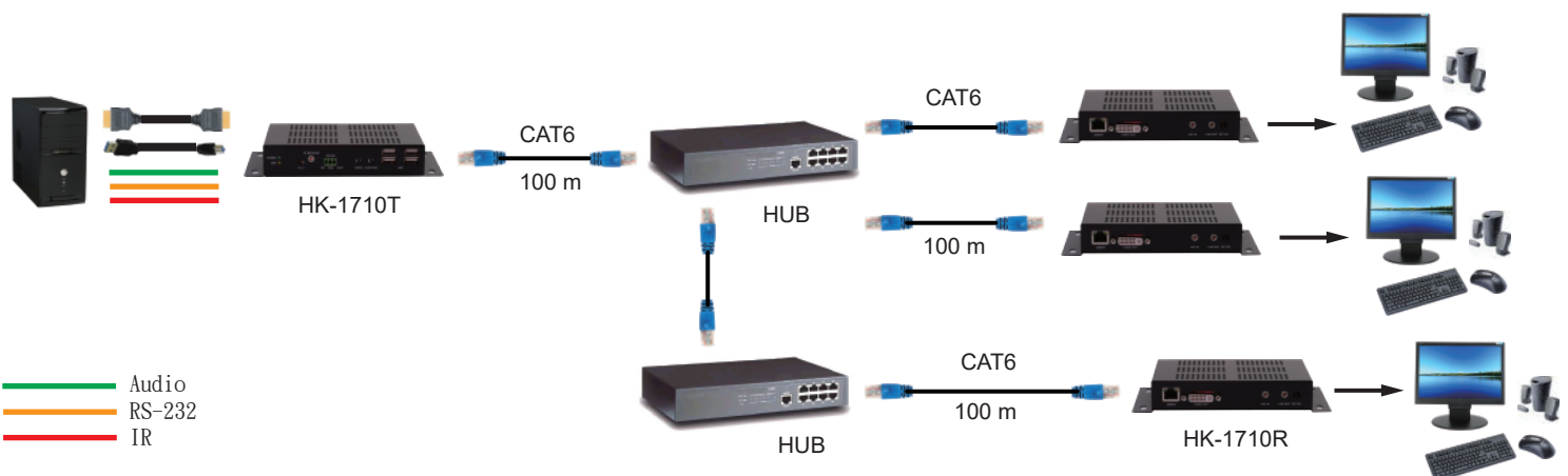
1對多 連接示意圖
